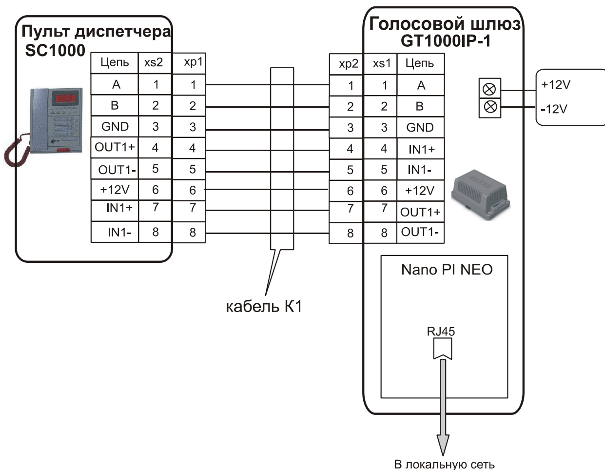
Рис.3 Схема подключения ГШ GT1000IP-1 к пульту диспетчера SC1000
